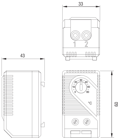
Thermostat NTL-10A
